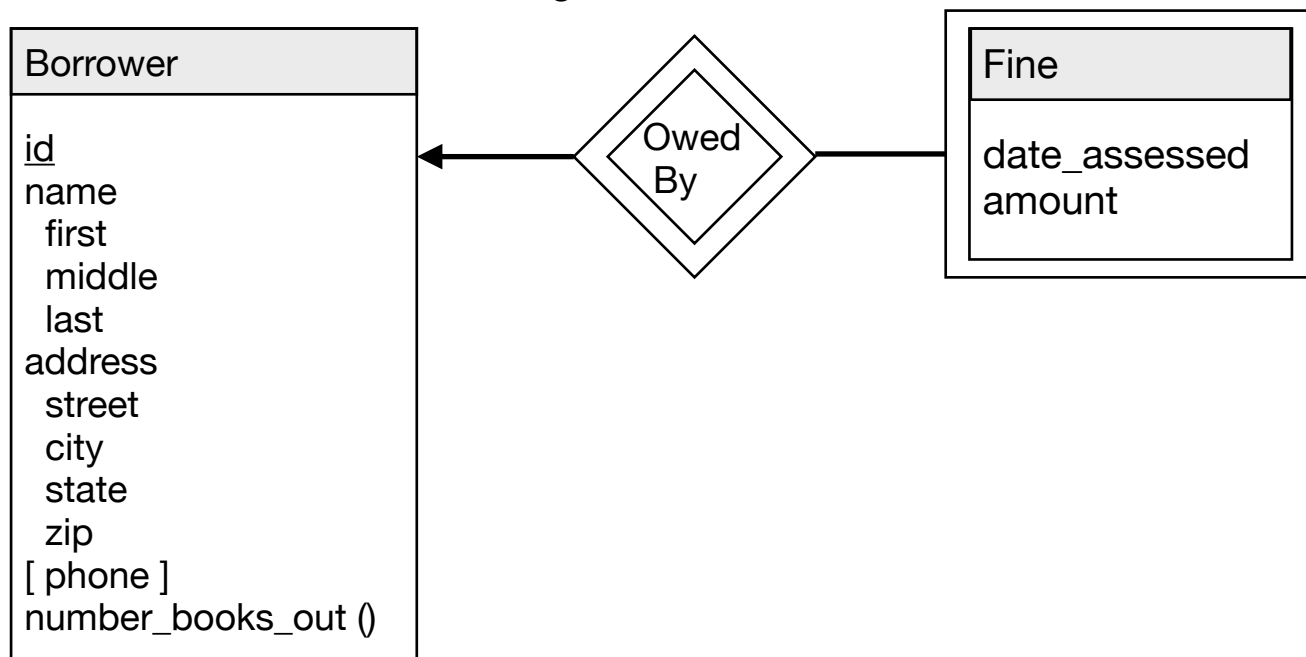
ER Diagram
